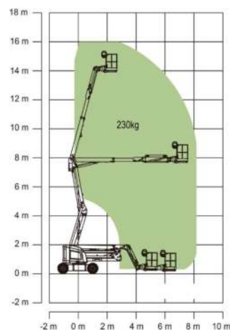
Rango de movimiento ZA14NJE/ZA14NJE-Li
